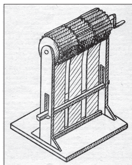
60 / Přístroj pro efekt střelby strojní puškou.
