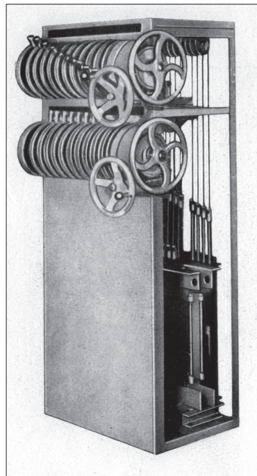
99 / První polovina 20. století byla provázena nástupem elektrického proudu na ochotnická jeviště. Jednosměrné stavědlo.
