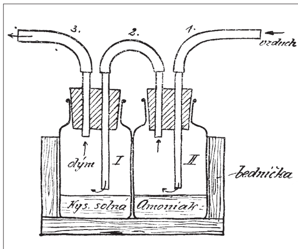
498 / Chemie ve službách ochotnického divadla. Přístroj na tvoření dýmu na jevišti z 20. let 20. století.
