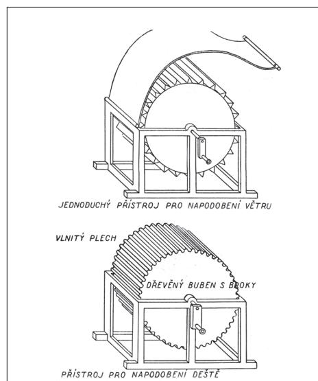
592 / Nedílnou součástí Kursu pro divadelní ochotníky vydaného 1942 byly přístroje napodobující zvuky.
