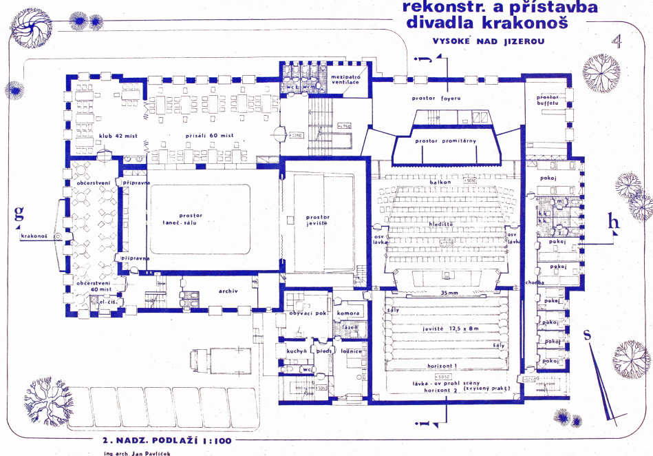
Vítězný návrh Jana Pavlíčka - půdorys 2. podlaží
