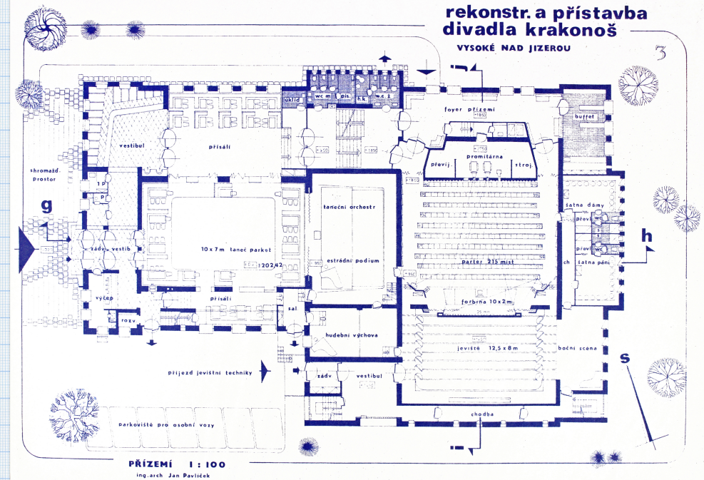
Vítězný návrh Jana Pavlíčka - půdorys přízemí
