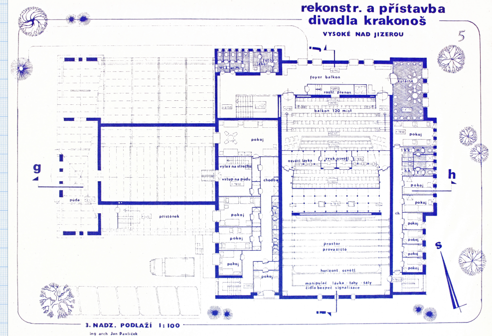
Vítězný návrh Jana Pavlíčka - půdorys 3. podlaží
