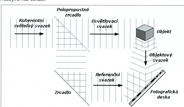
Záznam hologramu
