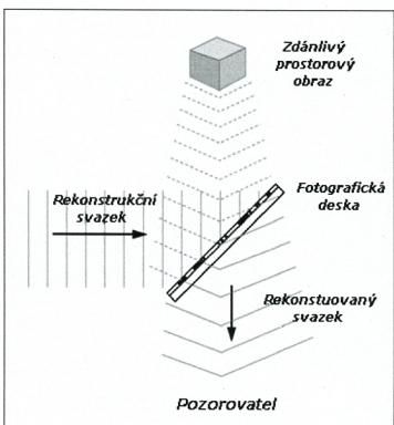
Rekonstrukce hologramu
