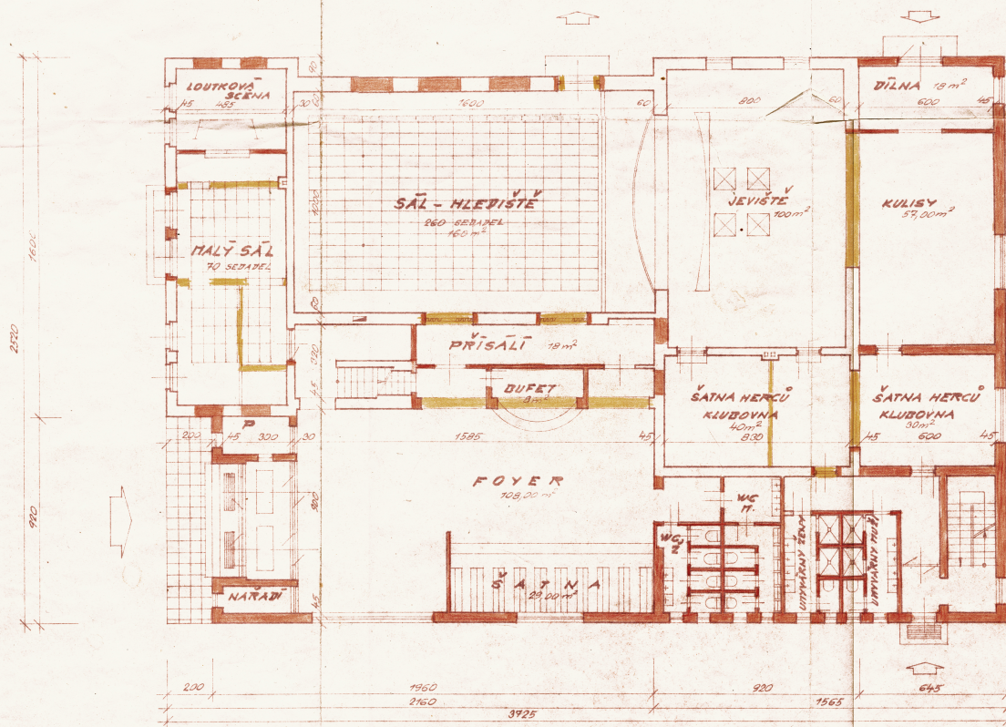
Návrh Jaroslava Pavla z roku 1970 - půdorys přízemí, boční řez a srovnání projektu s normou ČSN
