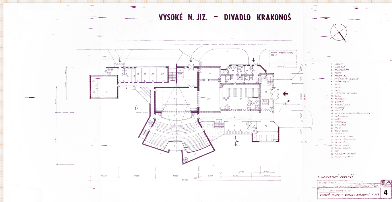
Návrh Karla Rulíka z roku 1989 - půdorys přízemí
