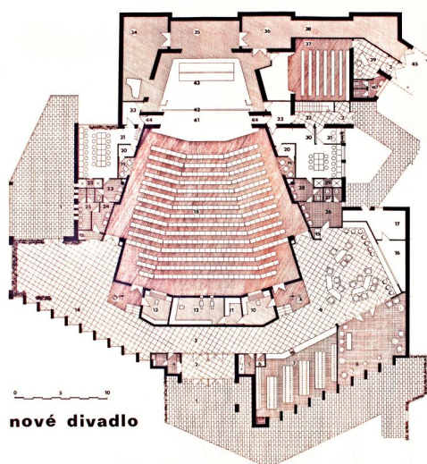
Varianta Dvojče - půdorys
