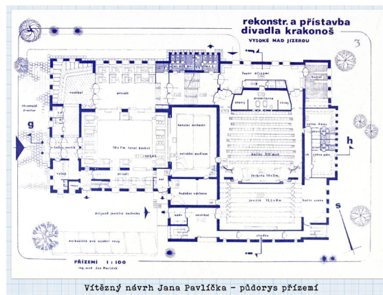
Vítězný návrh Jana Pavlíčka - půdorys přízemí
