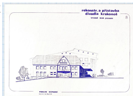
Vítězný návrh Jana Pavlíčka - pohled od západu (průčelí od kostela)
