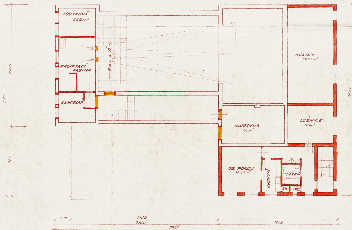
Návrh Jaroslava Pavlů z roku 1970 - půdorys 1.-3. patra a pohled od jihu (od hasičny)
